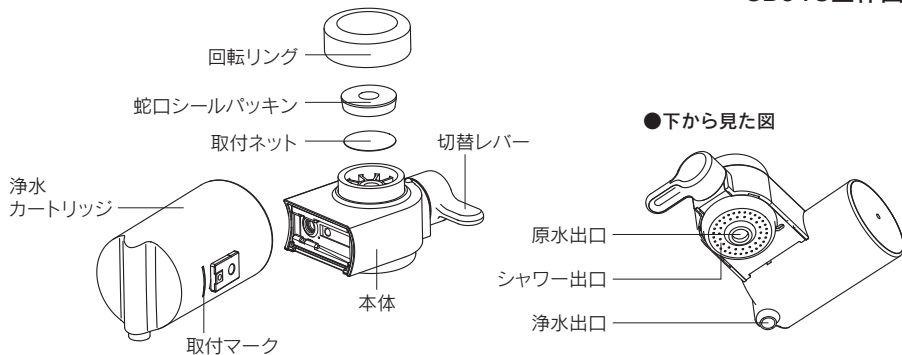
CB073全体図
