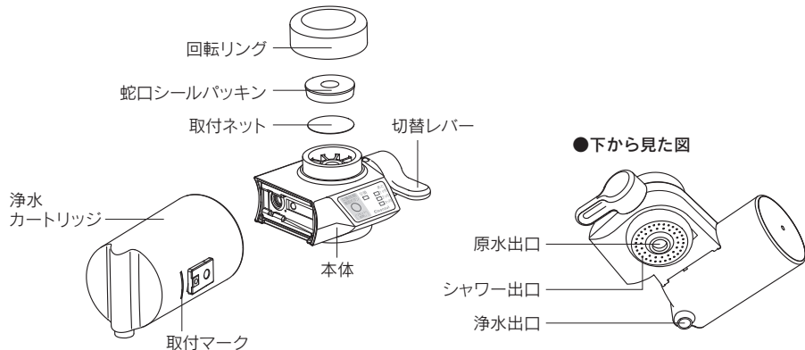
CB083全体図
